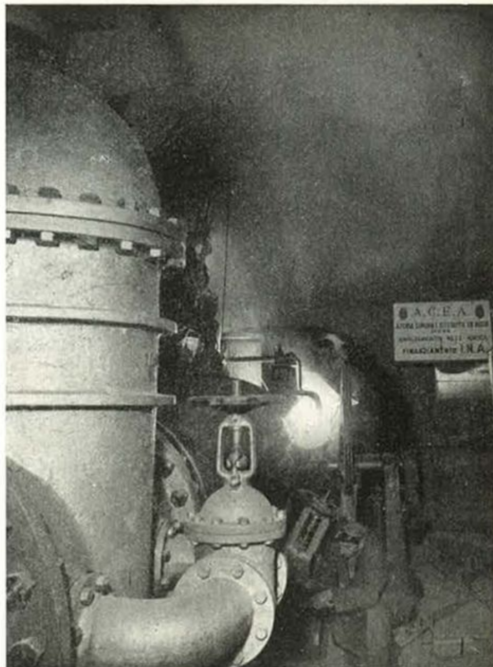
Acquedotto del Peschiera: attraversamento della depressione tiberina: particolari della valvola a farfalla «Calzoni» e della saracinesca «Breda».
