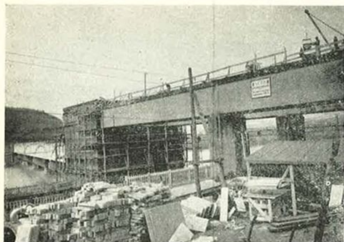
Esterno dei cunicoli di sinistra in cemento armato, per l'attraversamento della Ferrovia e del fiume Tevere.
