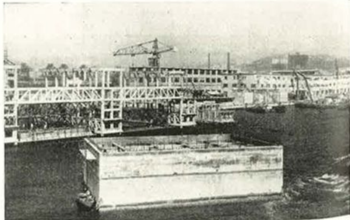
Cantiere a Ponte Canepa per la costruzione dei cassoni per la diga di protezione dell'aeroporto - Uno dei giganteschi cassoni già varato
