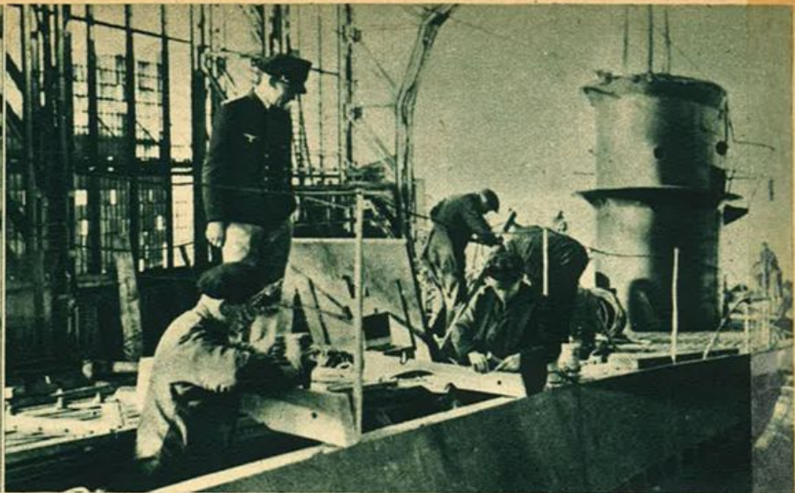
Sul sommergibile quasi ultimato viene costruito il ponte.
