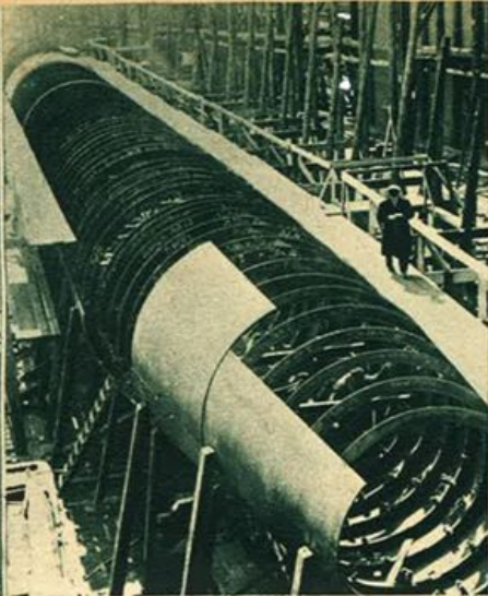
Un nuovo sommergibile sta prendendo corpo.
